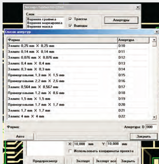
Апертурный лист
