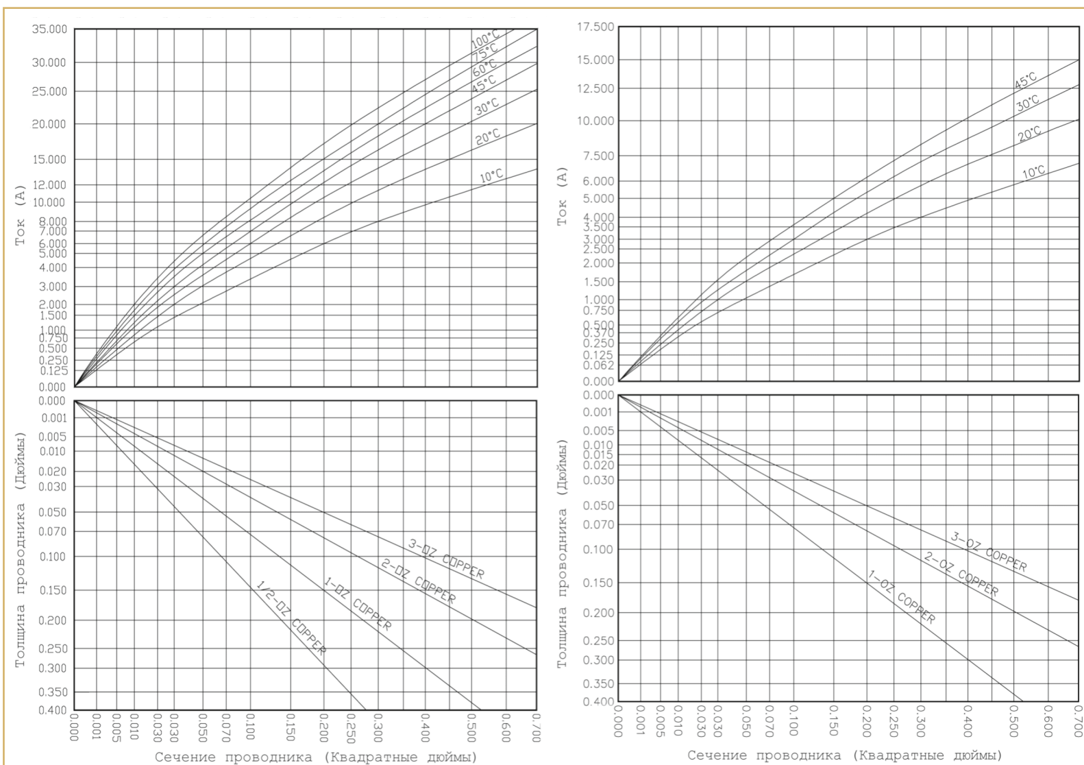
Выбор ширины и толщины проводников ПП в зависимости от силы тока: внешние слои
